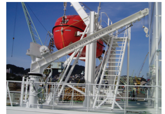
燃料ホース及びプロビジョンハンドリングクレーン (0.9TON×4.15MR) F.O.Hose handling & provision handling crane
