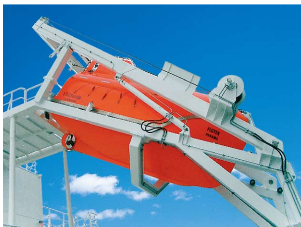
フリーホールランチングシステム Free-fall launching system
